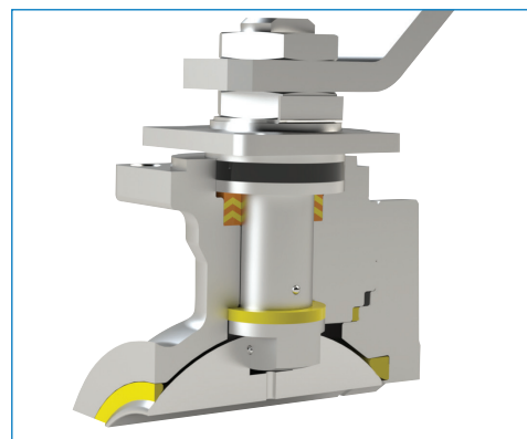
Sezione di valvola con pacco di tenuta asta provvisto di V-Pack - Valve section with V-Pack stem seal.
