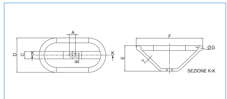
Volantino ovale per valvole flangiate e filettate - Oval handle for flanged and threaded ball valves - Oval handle pour taraudée Vanne à boisseau sphérique - Oval handle für kugelhähne mit gewinde - oder flanschanschluss - Oval handle por válvula de bola roscada o bridada.
