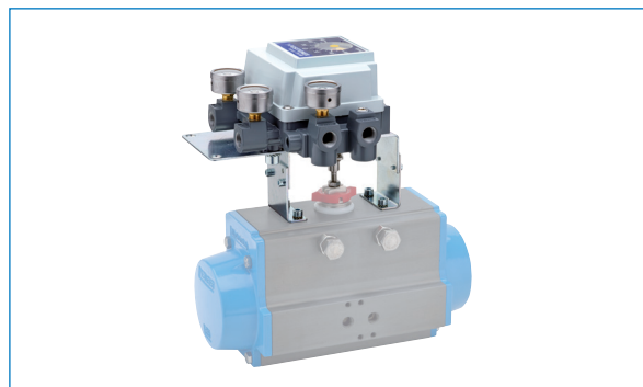
Attuatore pneumatico Valbia con posizionario - Valbia pneumatic actuator with positioner.
