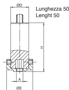
Prolunga per isolamento termico/coibentazione L50 - Thermal protection extension L50 - Extension pour isolation de calorifugeage L50 Spindelverlängerung für isolierte Rohrleitungen L50 - Elongador para aislamiento termico L50
