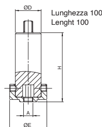
Prolunga per isolamento termico/coibentazione L100 - Thermal protection extension L100 - Extension pour isolation de calorifugeage L100 Spindelverlängerung für isolierte Rohrleitungen L100 - Elongador para aislamiento termico L100
