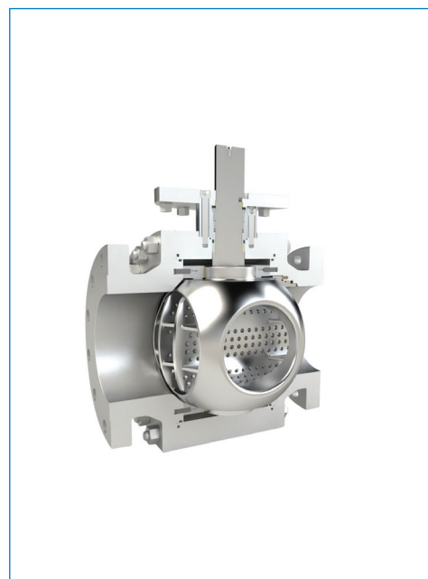
Sezione di valvola di regolazione per fluidi gassosi dotata di sfera con piastre forate - Example of gas fluid regulation valve: special trim ball section.
