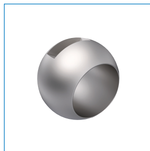
Sfera a passaggio totale per valvola flottante - Full bore ball valve, floating design.
